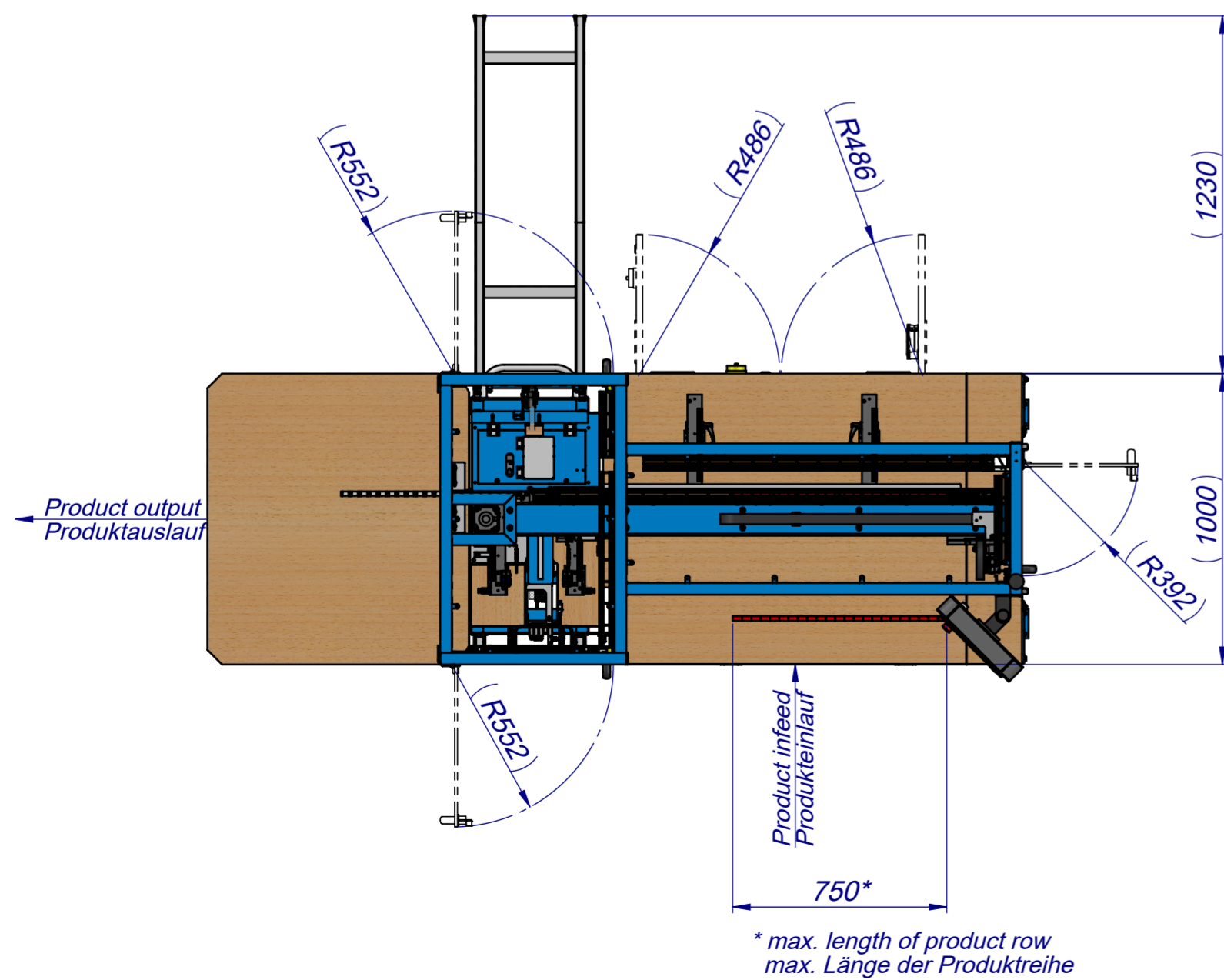
View without upper protection covers Ansicht ohne obere Schutzabdeckungen
